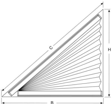
SDP2: Breite, Höhe, Schräge
