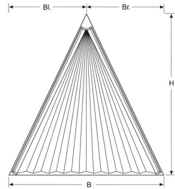
SD3: Breite, Höhe, Schräge links, Schräge rechts
